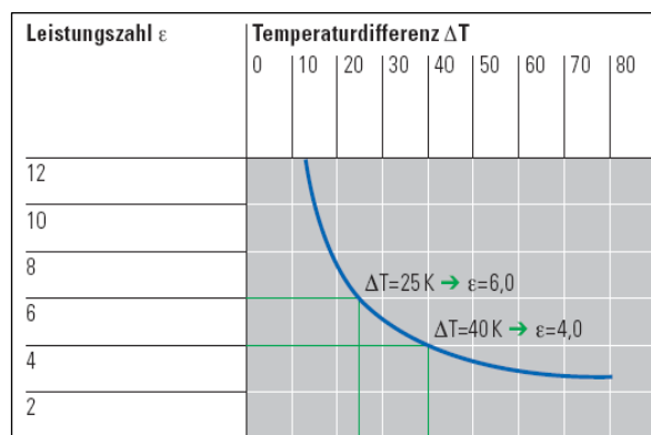
Abbildung 9: Leistungsanzahl \epsilon als Funktion der Temperaturdifferenz \Delta T zwischen Verdampfer und Verflüssiger ( T_0 = 273 \text{ K} ).
