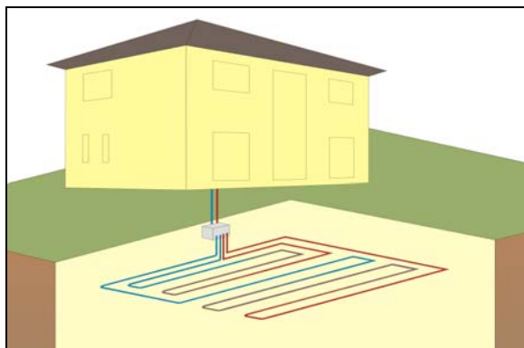
Abbildung 5: Schema Erdwärmekollektor
