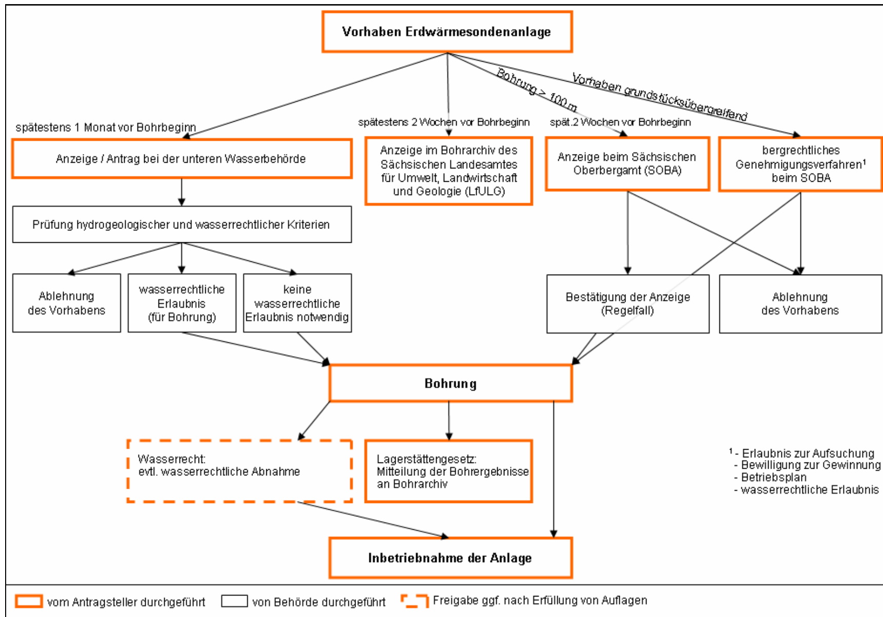
Abbildung 11: Ablaufschema Vorhaben Erdwärmesondenanlage.
