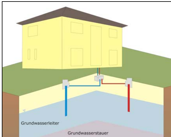
Abbildung 7: Schema Entnahme- und Einleitbrunnen.
