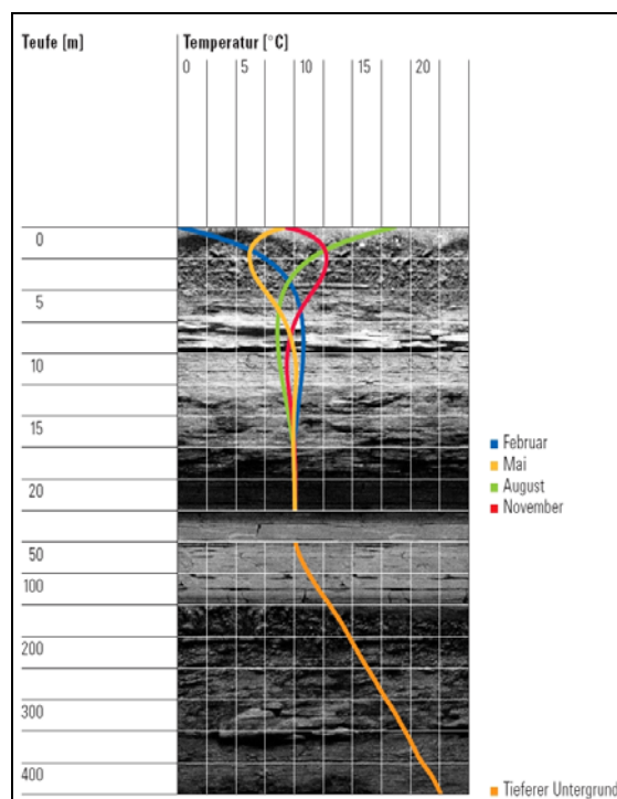
Abbildung 1: Temperaturverlauf in den oberen Bodenschichten.
