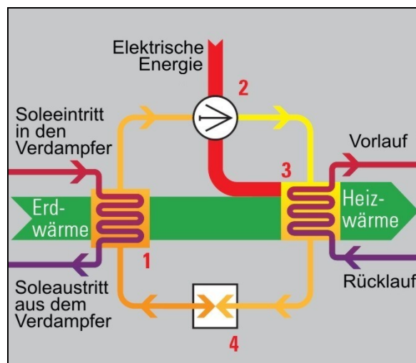
Abbildung 10: Funktionsprinzip einer Sole/Wasser-Wärmepumpe.
