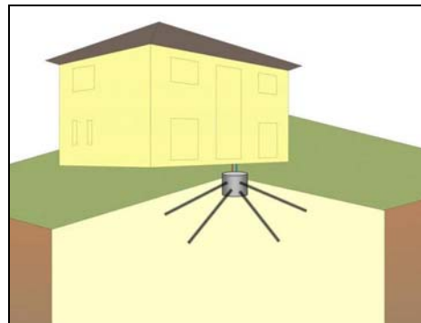
Abbildung 4: Schema schräge Erdwärmesonden nach GRD ® -Verfahren.
