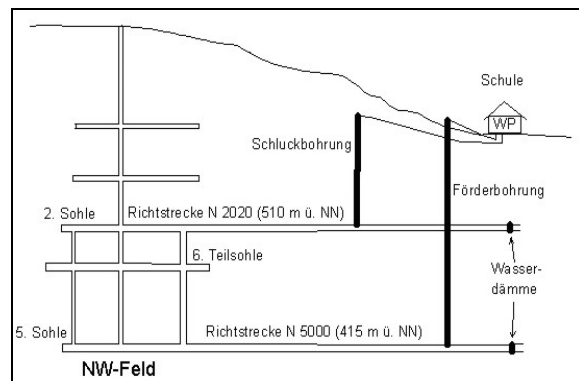
Abbildung 8: Schema Grubenwassernutzung der Zinngrube Ehrenfriedersdorf für die örtliche Mittelschule.
